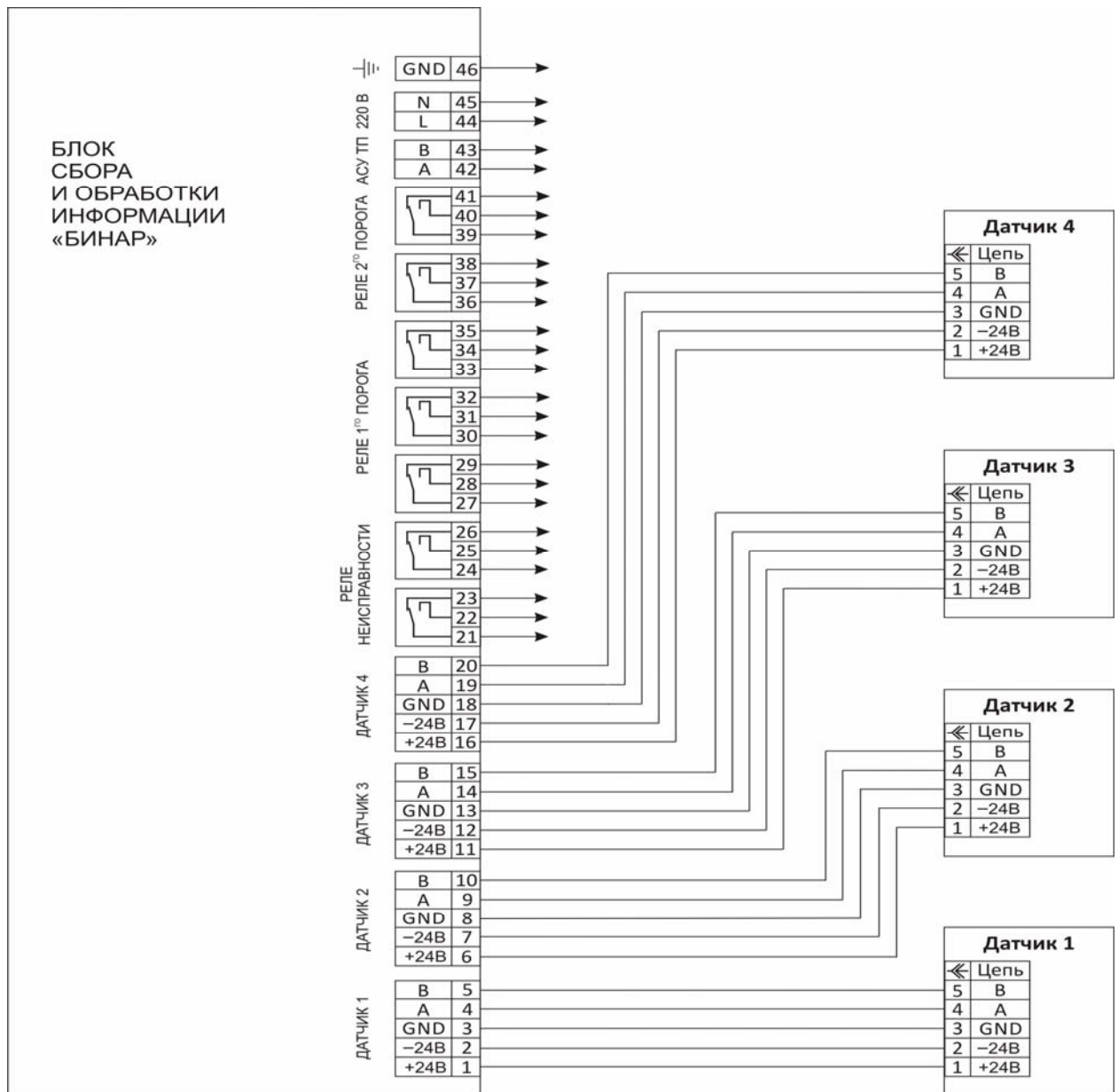
Рисунок №7 Схема электрическая
