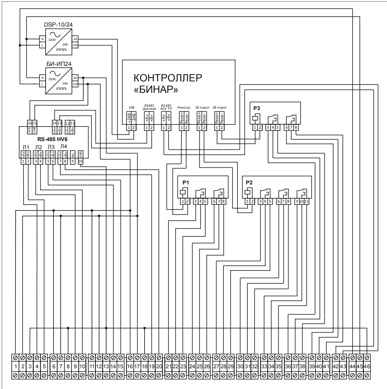
Рисунок №6 Схема межблочных соединений
