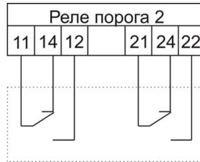
Состояние контактов реле Порога 2, когда установленный порог превышен
