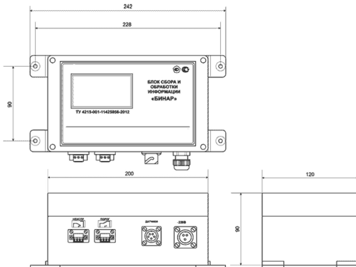
Рисунок №1 Настенный моноблок БСИ "Бинар"
