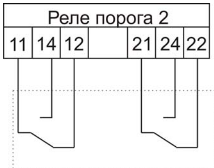
Состояние контактов реле Порога 2, когда установленный порог не превышен
