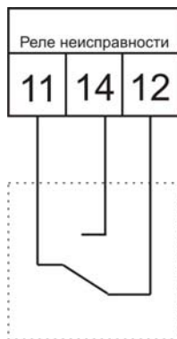
Состояние контактов реле при неисправности
