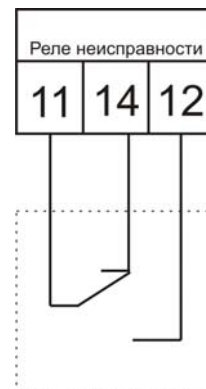
Состояние контактов реле при нормальном режиме
