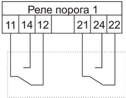
Состояние контактов реле Порога 1, когда установленный порог не превышен
