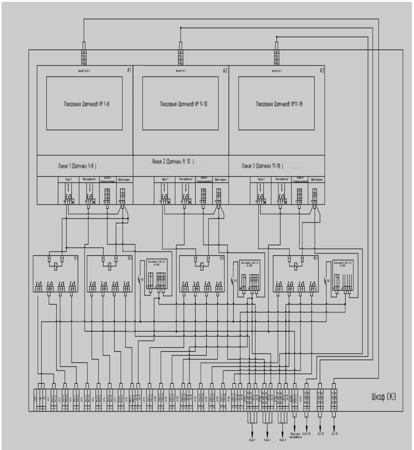
Рисунок №3 Схема межблочных соединений
