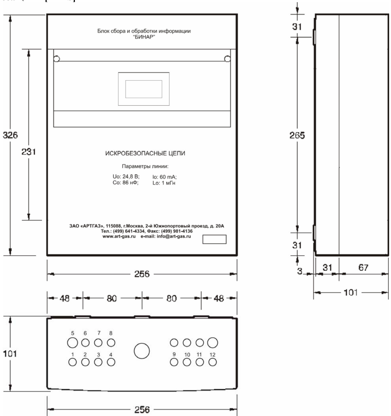
Рисунок №5 Модульное исполнение в электромонтажном шкафу
