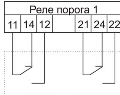
Состояние контактов реле Порога 1, когда установленный порог превышен
